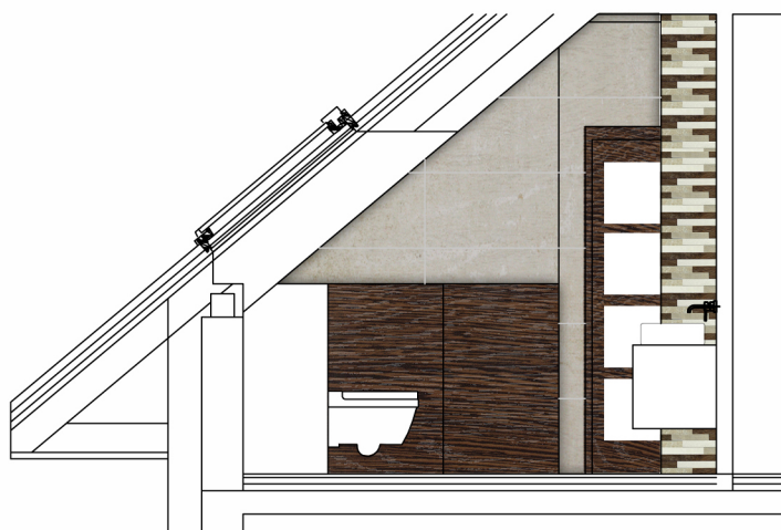
widok C/1:50
