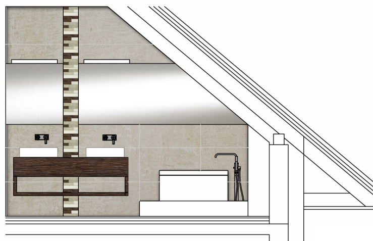
widok D/1:50
